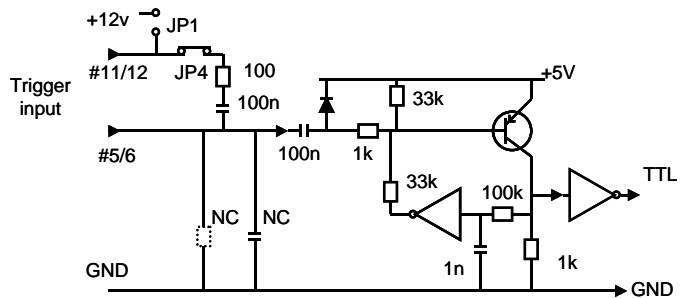
Fig. 5. Trigger input.
